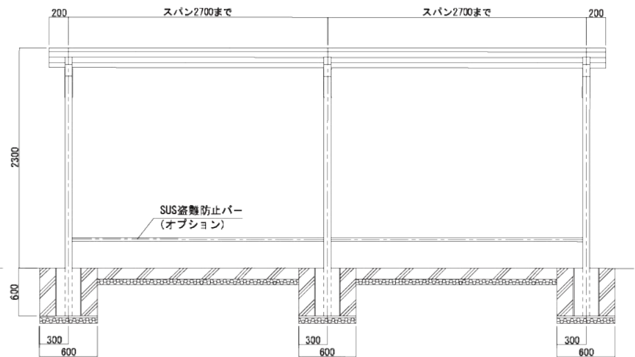
立面図
